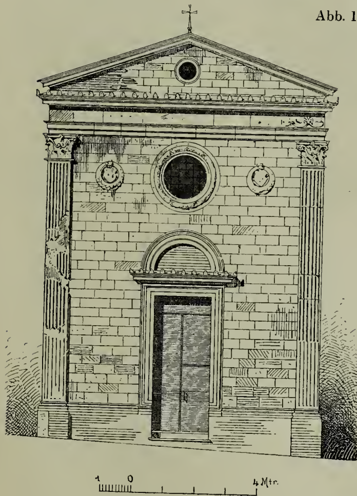
Abb. 128. S. Maria delle nevi zu Siena. (Gnauth.)
